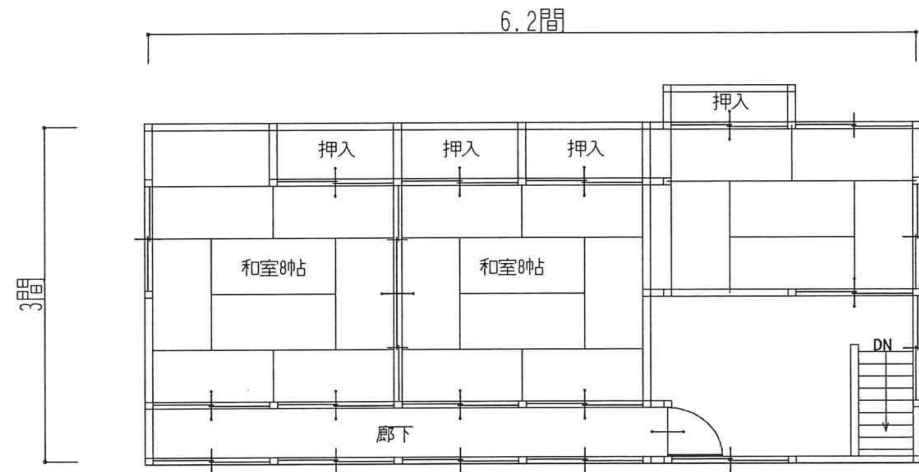
<2階>
